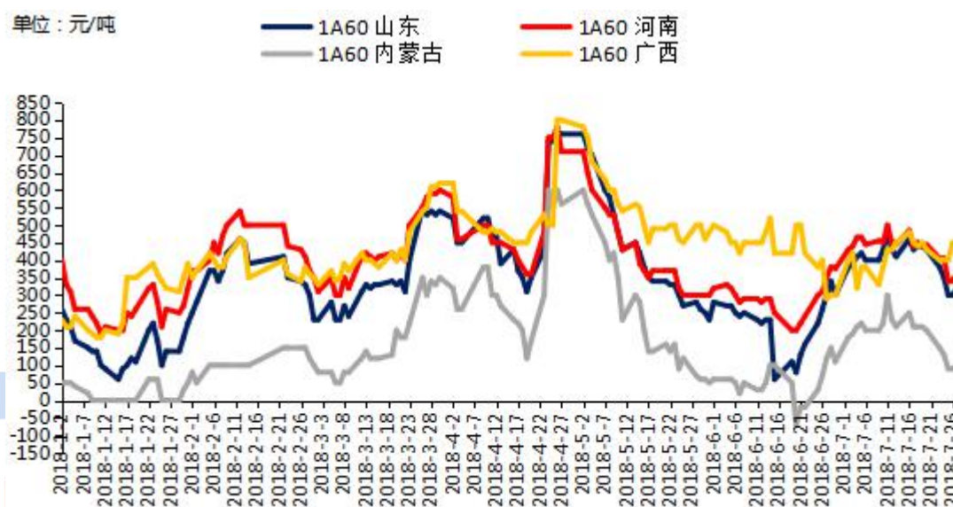
图 1. 2016-2018 年全国主流地区 1A60 电工圆铝杆价格走势
