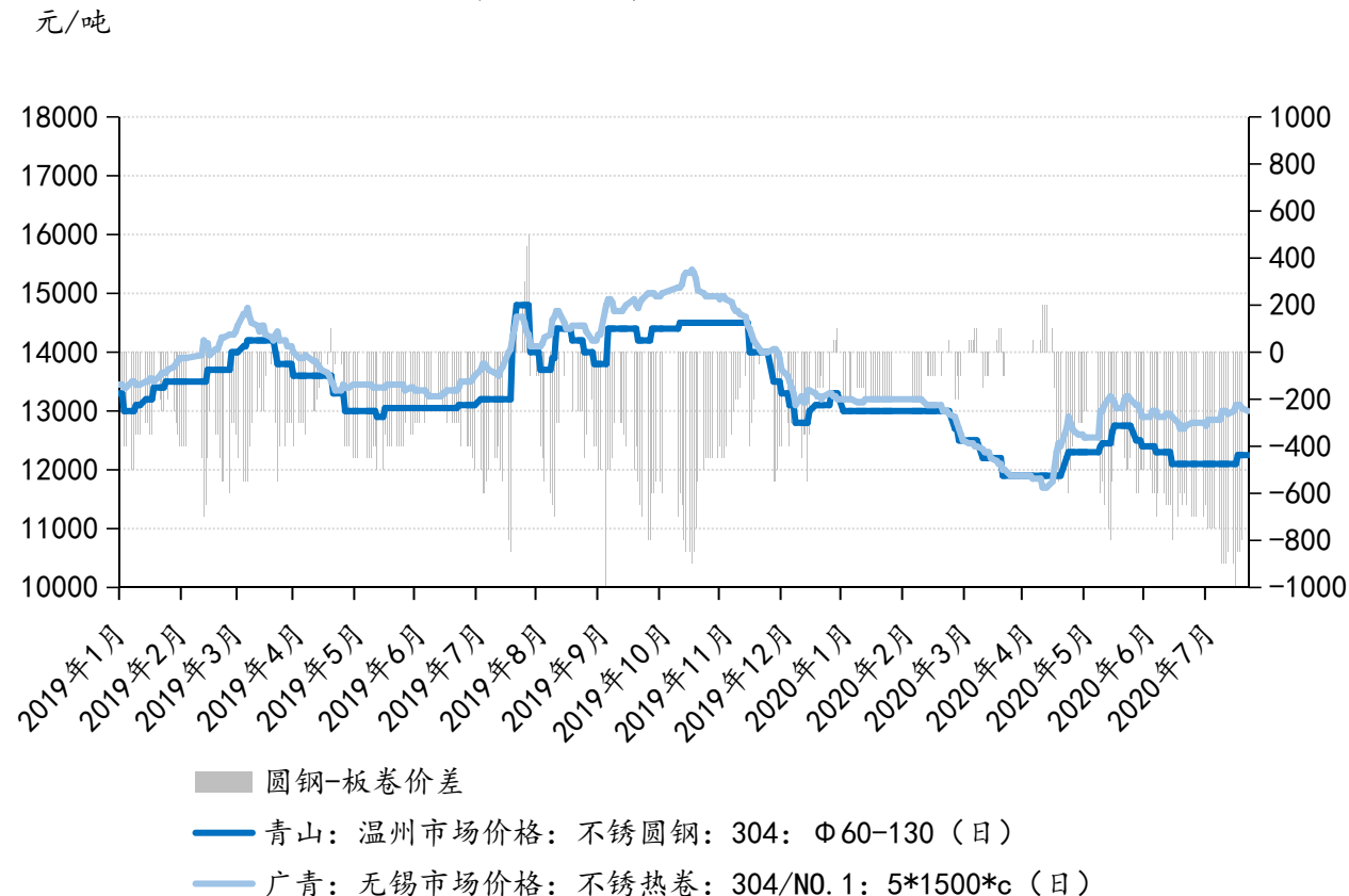
300系不锈钢棒材与板卷价格对比
