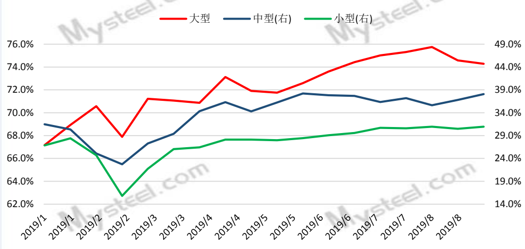
Mysteel统计国内矿山分规模产能利用率
