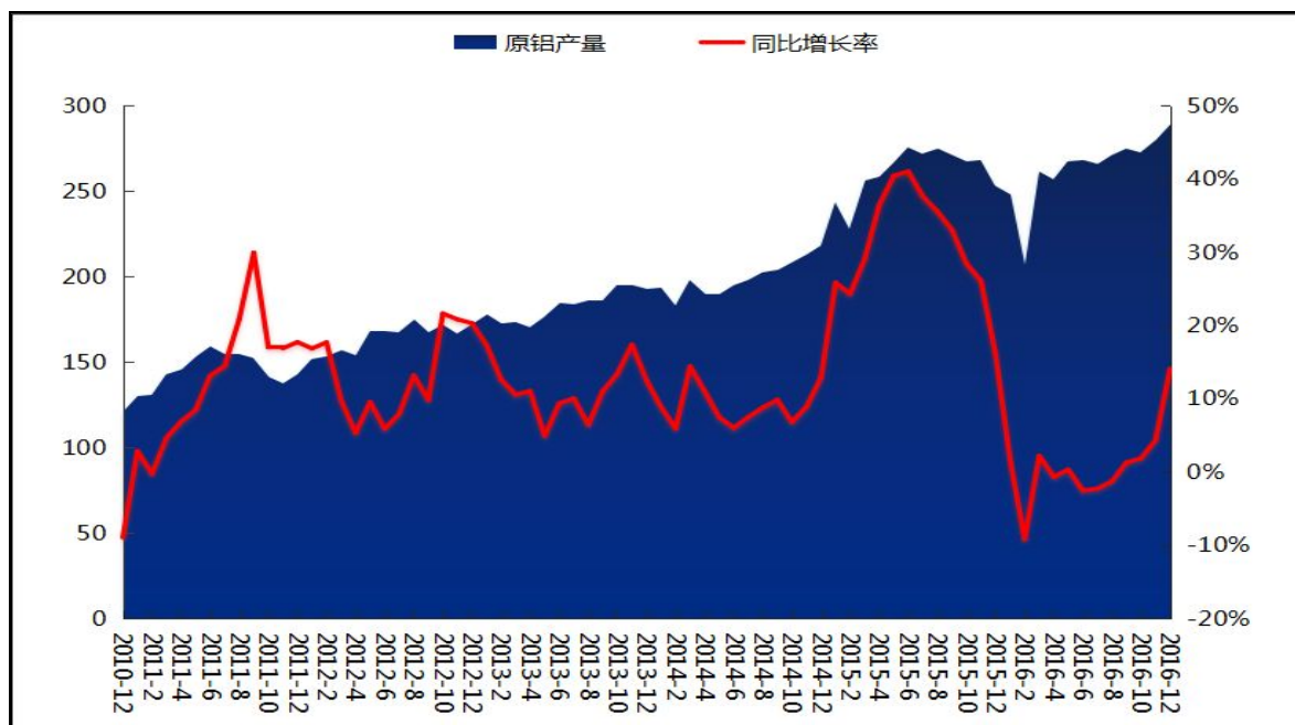
图 9、2016年12月国内电解铝产量图（万吨）
