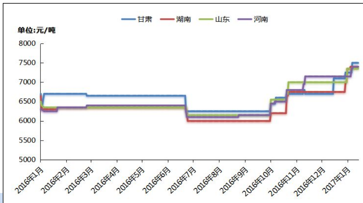
图 15、12月份国内主流地区氟化铝参考报价
