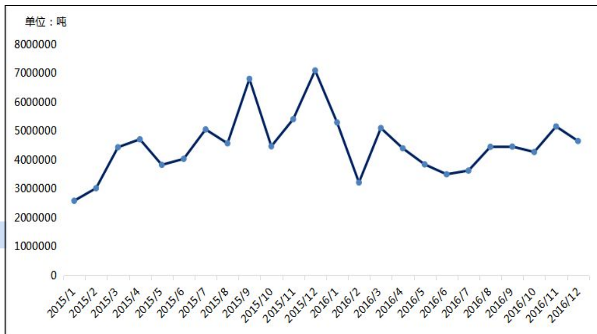
图 1、2015 年 1 月至 2016 年 12 月中国进口铝土矿月度总量(吨)
