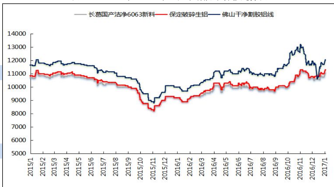
图 25、2015年-2017年主流市场废铝价格走势
