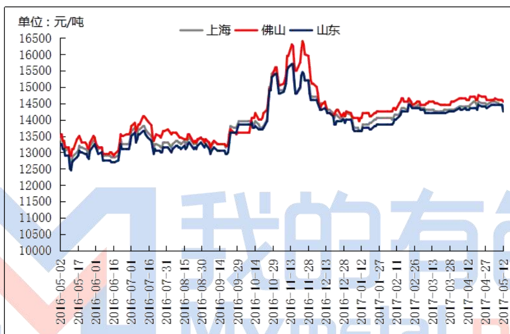
图4. 全国主流地区 A356.2 铝合金锭价格走势 规格：国标
