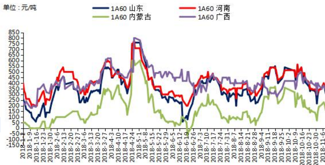
图 1. 2016-2018 年全国主流地区 1A60 电工圆铝杆价格走势
