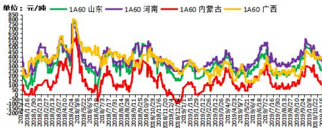
图 1. 2018-2019 年全国主流地区 1A60 电工圆铝杆价格走势图
